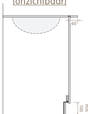
Afschroefbaar paneel (onzichtbaar)
