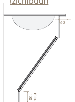
Afschroefbaar paneel (zichtbaar)
