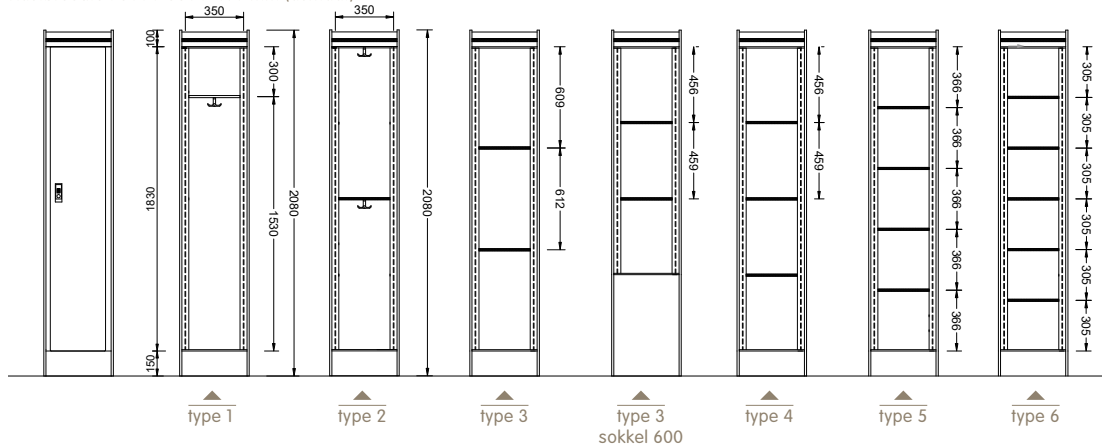
Kastbreedte : 300 / 350 / 400 mm (asmaat)
